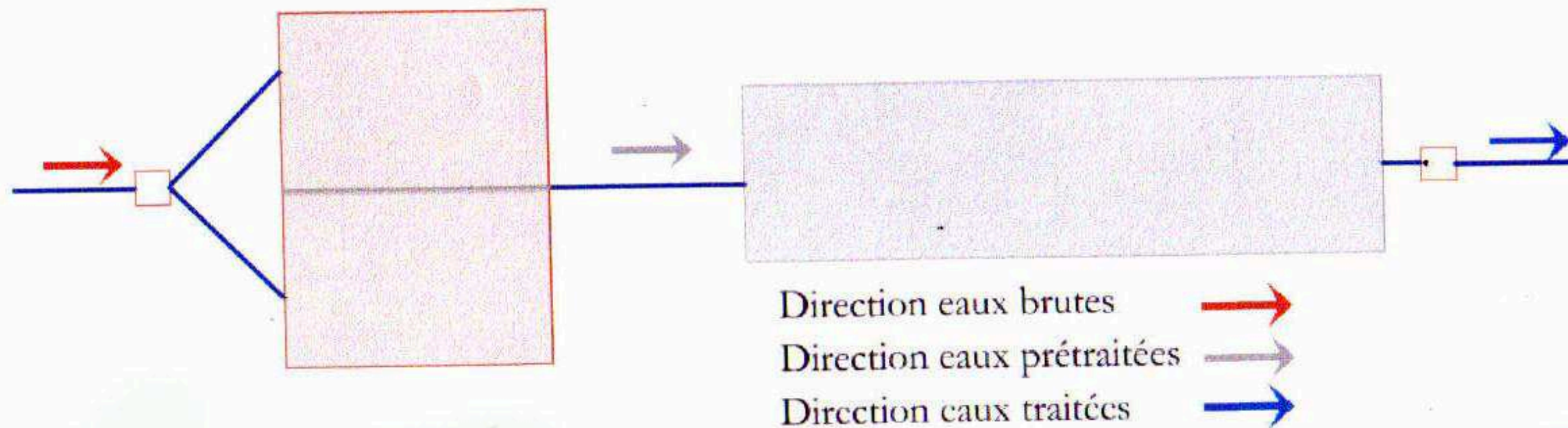
Filtre vertical
